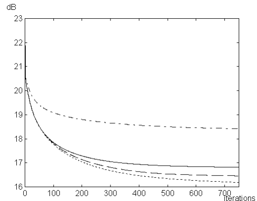
Fig. 5 10 \cdot \log_{10}(\epsilon^2 / \|n\|^2) :
